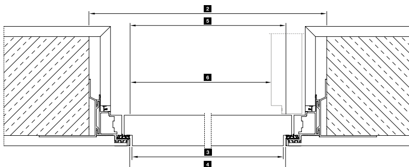
Vodorovný řez s dveřním křídlem s reverzním otevíráním
