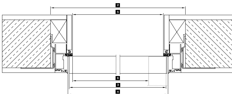
Vodorovný řez křídlem dveří s dorazem natupo
